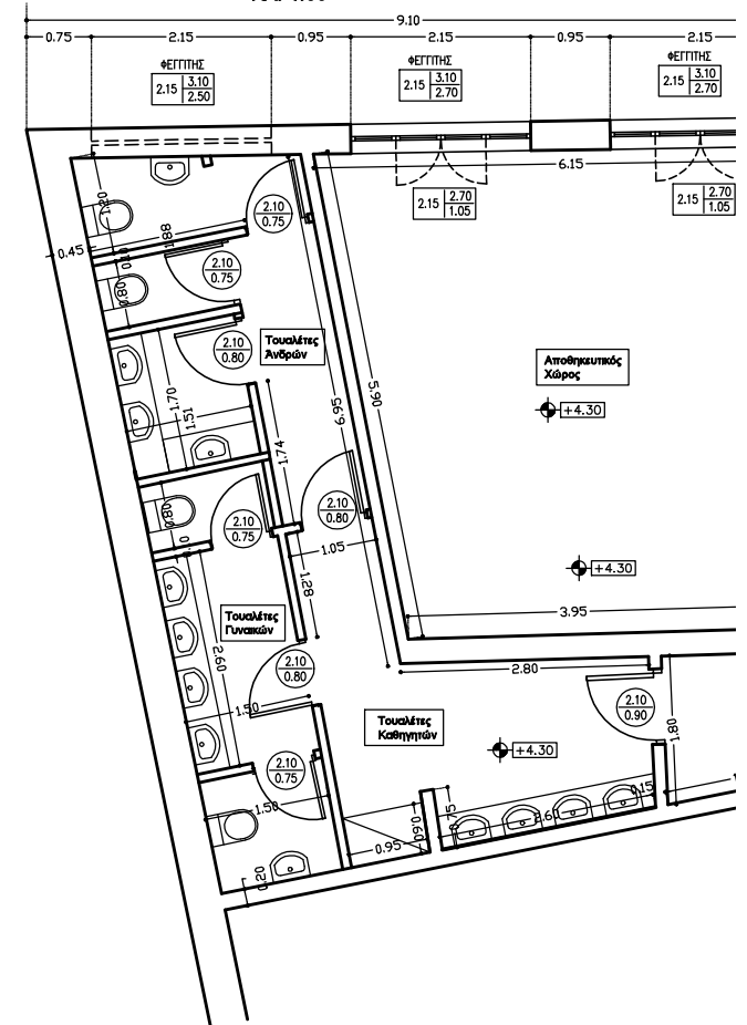
ΤΟΥΛΕΤΕΣ ΚΑΘΗΓΗΤΩΝ ΠΡΟΒΛΕΠΟΜΕΝΗ ΚΑΤΑΣΤΑΣΗ ΚΛ. 1:50
